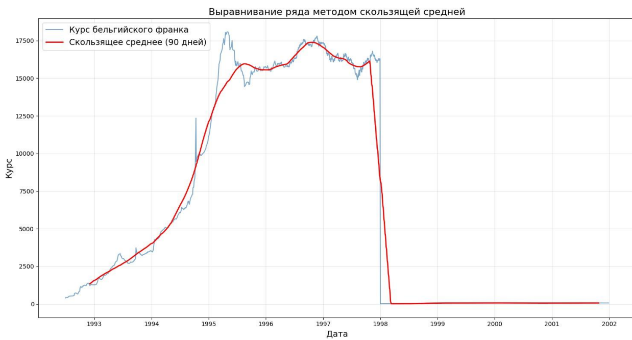
Рис. 23 Выравнивание ряда методом скользящей средней (окно 90 дней)
